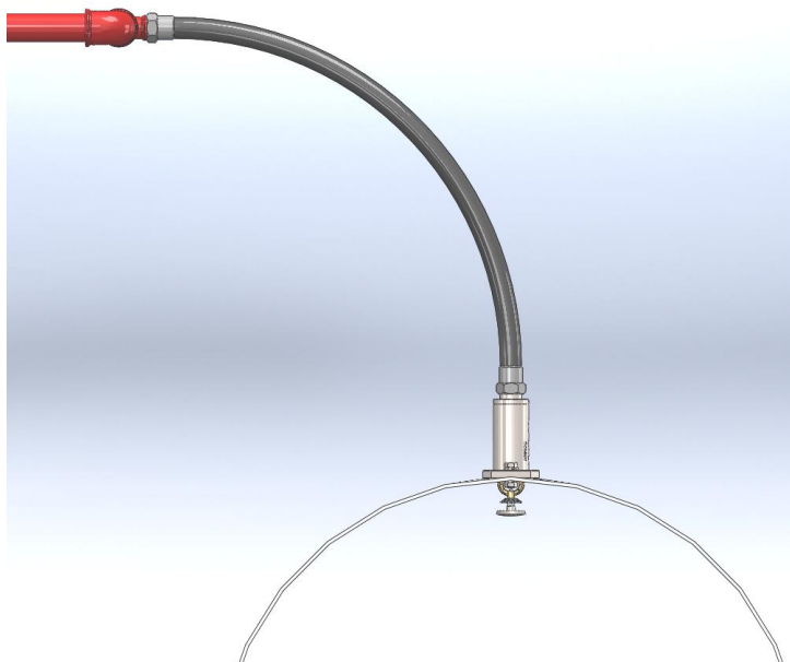
Rys. 4 Zraszacz ZS-15/O z podstawą prostokątną do montażu na kanałach okrągłych.
